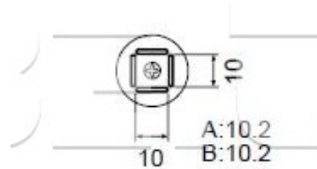
A1125B QFP 10 x 10
