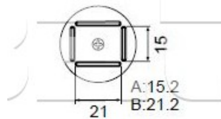
A1128B QFP 14 x 20
