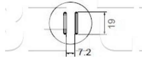
A1134 SOP 7.5 x 18
